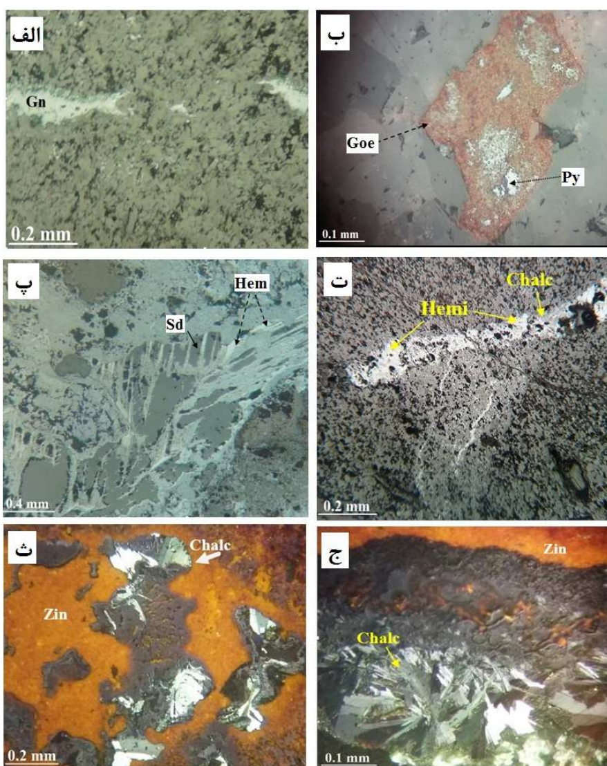
شکل ۶ الف) گالن به صورت رگه‌ای در زمینه‌ای از کربنات‌ها (نور بازتابی، PPL). ب) جانشینی کانه پیریت توسط گوتیت؛ (نور بازتابی، PPL). پ) هماتیت در راستای رخ‌ها جانشین کانی سیدریت شده است (نور بازتابی، PPL). ت) گسترش کانی‌های کالکوفانیت (خاکستری تیره و شعاعی) و همی‌مورفیت (خاکستری روشن) در زمینه‌ای از هیدروزینسیت (نور بازتابی، PPL). ث) گسترش کانی کالکوفانیت با بافت تیغه‌ای و پرکننده فضای خالی در زمینه‌ای از کانی هیدروزینسیت (نور بازتابی، XPL). ج) کالکوفانیت با بافت تیغه‌ای به همراه هیدروزینسیت؛ (نور بازتابی، XPL). د) گالن، Py: پیریت، Gth: گوتیت، Hem: هماتیت، Sd: سیدریت، Chal: کالکوفانیت، Hemi: همی‌مورفیت، Zen: هیدروزینسیت [۱۲].
