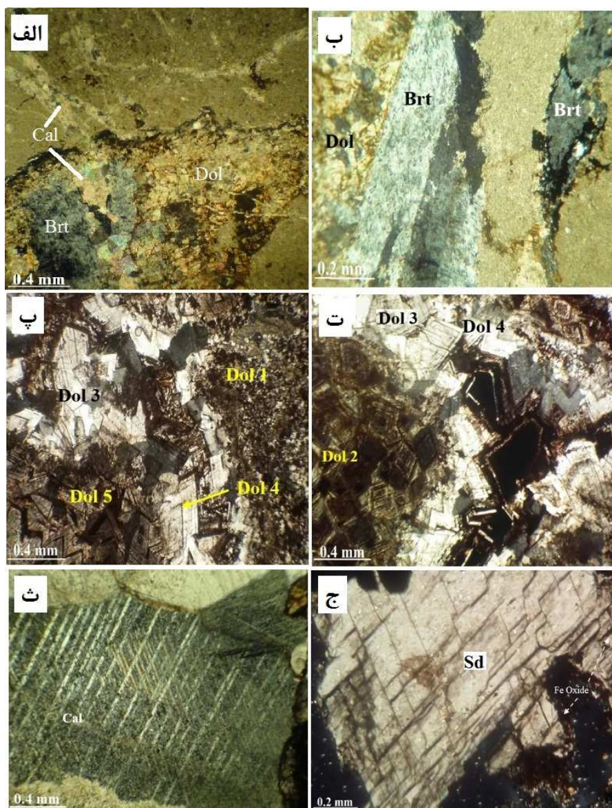
شکل ۵ الف) باریت با بافت دانه‌ای نیمه شکل‌دار تا کشیده در پهنه کانسنگ یال شرقی (نور عبوری قطبیده متقاطع، XPL). ب) باریت تیغه‌ای درشت بلور با ماکل کارلسباد در کنار دولومیت (نور عبوری، XPL). پ) و ت) نسل‌های مختلف کانی دولومیت در سنگ میزبان (نور عبوری، XPL). ث) کلسیت درشت بلور در کانسنگ (نور عبوری، XPL). ج) سیدریت که در راستای رخ‌های لوزی رخ خود به اکسیدهای آهن تجزیه شده است (نور عبوری قطبیده صفحه‌ای، PPL). باریت: Brt، دولومیت: Dol، کلسیت: Cal، سیدریت و Fe Oxide: اکسیدهای آهن [۱۲].
