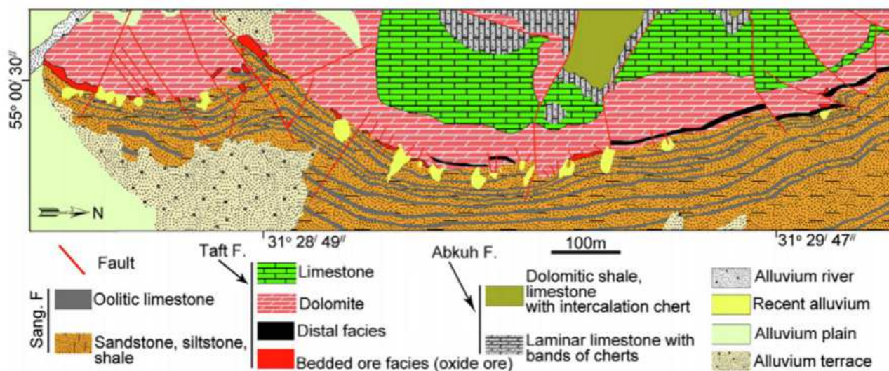
شکل ۳ نقشه زمین‌شناسی بخش کانسانگ یال شرقی کانسانر مهدی‌آباد که نشان‌دهنده موقعیت کان‌تن‌ها در مرز سازند تفت و سنگستان است [۹].
