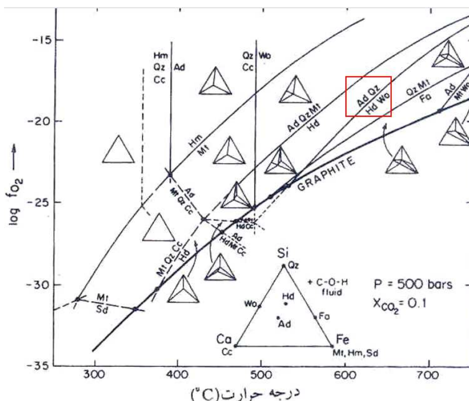
شکل ۱۱ نمودار سامانه Ca-Fe-Si-C-O-H و تعیین شرایط دمایی در برون‌اسکارن‌های گنبدنمکی زندان. مربع نشان‌دهنده مجموعه کانیاپی، Ad: آندرادیت؛ Hd: هدنبرژیت؛ Qtz: کوارتز و Wo: ولاستونیت است [۲۰].
