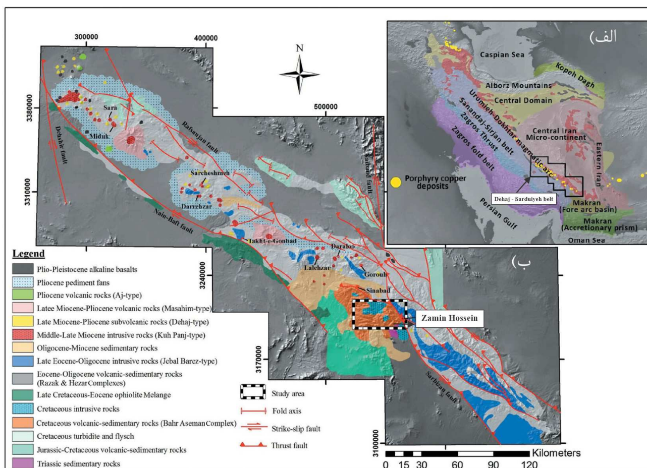
شکل ۱ (الف) پهنه‌های ساختاری ایران [۱] که در آن، موقعیت کمرند دهج-ساردوئیه (کمان ماگمایی سنوزوئیک کرمان، KCMA) و کمرند ماگمایی ارومیه-دختر نشان داده شده است. (ب) نقشه زمین‌شناسی ساده شده کمرند دهج-ساردوئیه که در آن موقعیت منطقه مورد بررسی و تعدادی از ذخایر مس پورفیری شناخته شده در ایران نمایش داده شده است (برگرفته از مرجع [۱۵] با کمی تغییرات).
