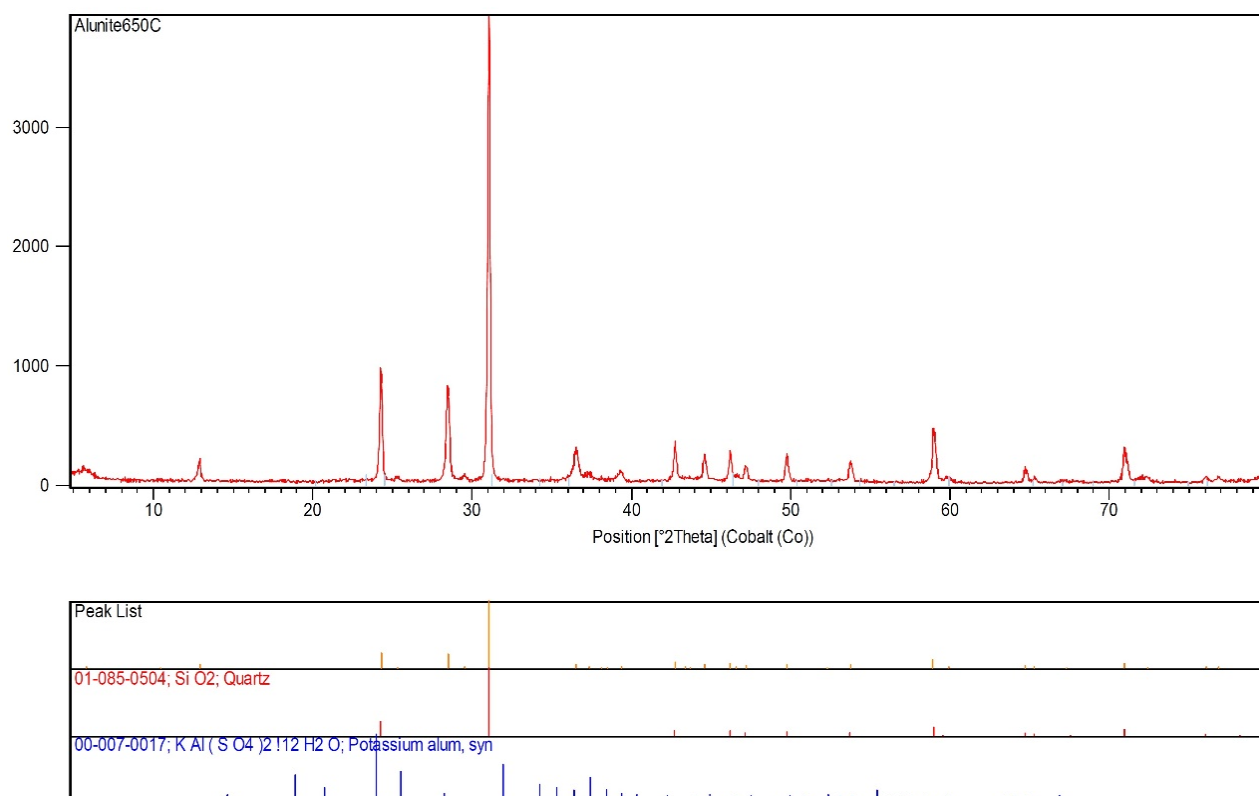
شکل ۹ طیف پراش پرتو ایکس نمونه پس از گرمادهی تا دمای ۶۵۰ درجه سانتیگراد که باعث آب‌زدایی آلونیت شده است.
