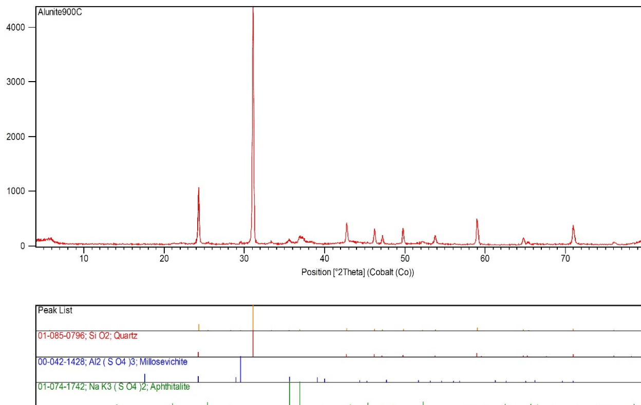
شکل ۱۰ طیف پراش پرتو ایکس نمونه پس از گرمادهی تا دمای ۹۰۰ درجه سانتیگراد که باعث تشکیل فاز آفتیتالیت \text{NaK}_3(\text{SO}_4)_2 شده است.
