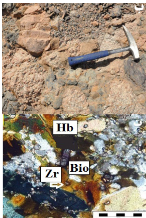
شکل ۴ الف - قطع‌شدگی سنگ‌های گنیسی میزبان توسط دایک‌های گرانیتی آپلیتی در غرب مغستان (شمال مجموعه نی‌باز، دید به سوی جنوب). ب - کنگلومرای قاعده کرتاسه در جنوب غرب ساغند که سرشار از قلوه‌های سنگی میکاشیستی، گنیسی، آمفیبولیتی، مرمری، گرانیتی و گابرویدیوریتی است. پ - تصویر میکروسکپی میکاشیست‌های چین‌خورده با بافت لپیدوبلاستی بارز. ت - تصویر میکروسکپی گنیس‌های بیوتیت‌دار سرشار از زیرکن. دگرشکلی مومسان از ویژگی بارز این سنگ‌هاست (هورنبلند سبز: Hb، بیوتیت: Bio، زیرکن: Zr)
