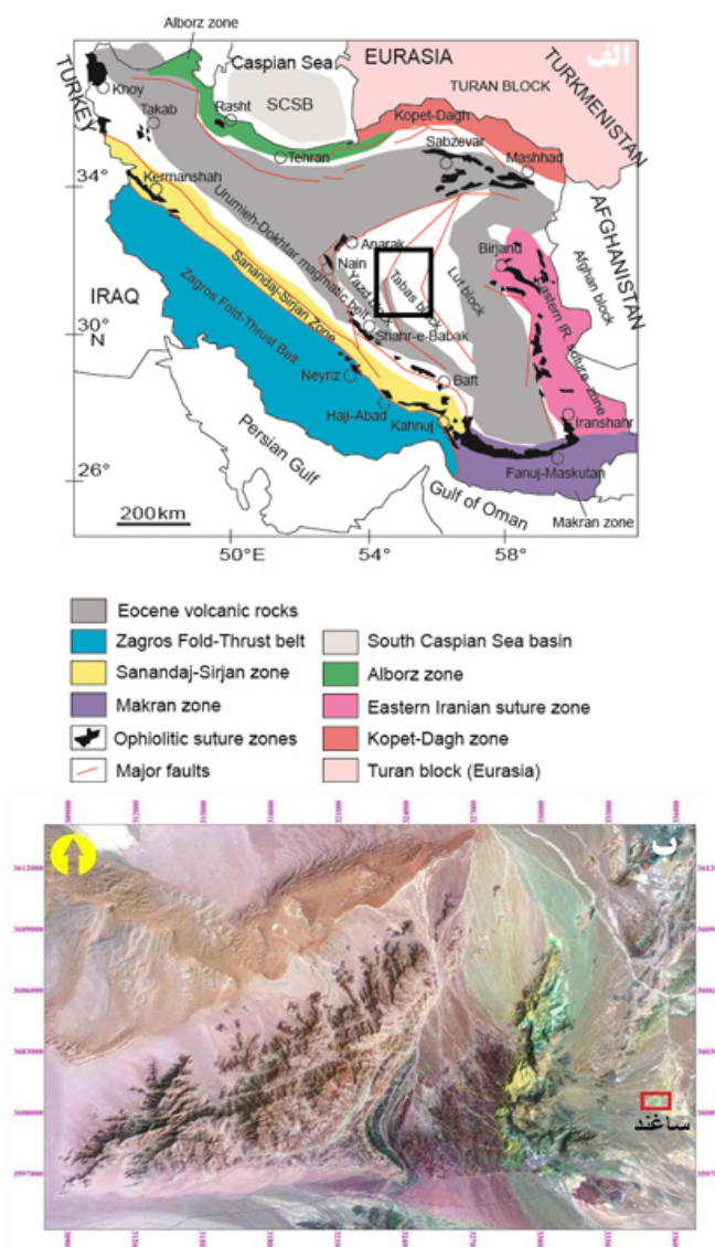
شکل ۲ الف- نقشه پهنه‌های ساختاری ایران و جایگاه تقریبی مجموعه نی‌باز (مستطیل مشکی) بر آن و ب- تصویر ماهواره‌ای نشان‌دهنده مجموعه دگرگونی - آذرین نی‌باز. دور تصویر بر حسب سیستم مختصات جهانی رکاتور معکوس UTM مدرج، است.
