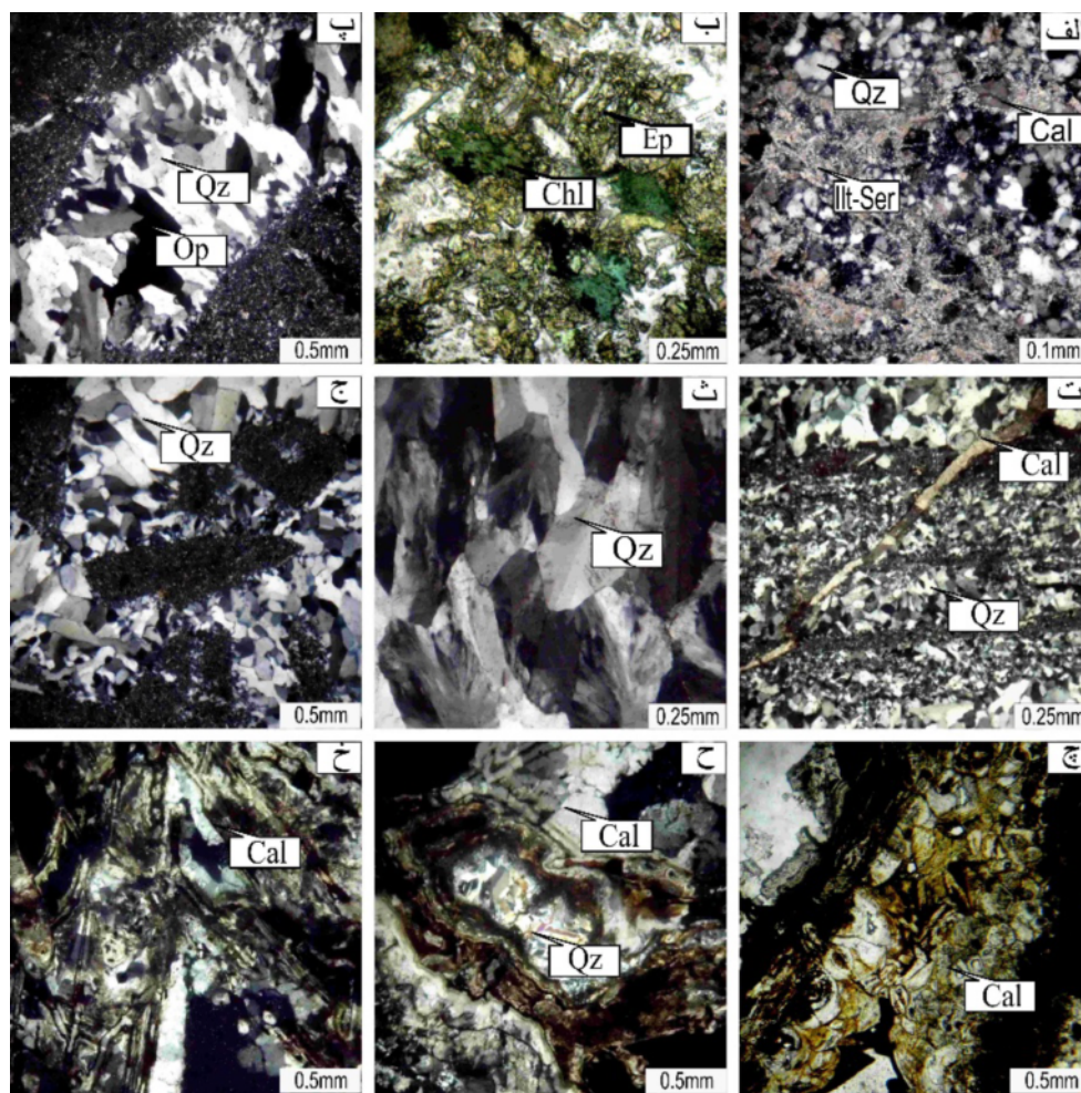
شکل ۴ الف) رخداد دگرسانی آرژیلیک حدواسط با توجه به حضور کانی‌های کلسیت (Cal)، ایلیت-سریسیت (Ill-Ser) و کوارتز (Qtz). (نور xpl)، ب: دگرسانی پروپلیتی با حضور اپیدوت (Ep) و کلریت (Chl). (نور ppl)، پ: رگه کوارتزی-سولفیدی با بافت شانه‌ای. (نور xpl)، ت: رگه کربناتی دربردارنده کوارتز با بافت قشرگون. (نور xpl) ث: بافت پرماند (باطله کوارتز). (نور xpl) ج: بافت برشی (قطعاتی از سنگ میزبان در یک زمینه سیلیسی). (نور xpl) چ: بافت گل کلمی به همراه رگه‌های کربناتی. (نور ppl) ح: بافت شانه‌ای و جانشینی کلسیت به جای کوارتز. (نور xpl) و خ: بافت تیغه‌ای به همراه رگه‌های کربناتی. (نور xpl).
