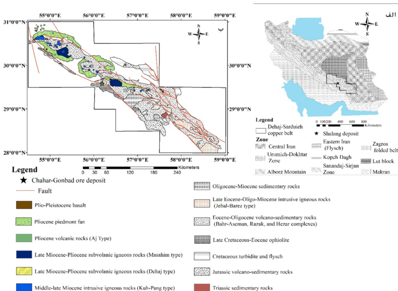
شکل ۱ الف: نقشه پهنه‌های ساختاری ایران و جایگاه کمر بند دهج-ساردوئیه بر کمان آتشفشانی-نفوذی ارومیه-دختر همراه با سنگ‌شناسی ساده شده کمر بند دهج-ساردوئیه (بر گرفته از مرجع [۵] با اندکی تغییرات) و جایگاه ذخیره شلنگ بر آن.
