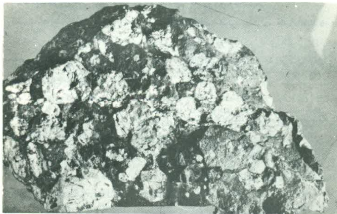
شکل ۱ درشت بلورهای آنالسیم در نقریتهای طالقان، مقیاس طبیعی است. به انکلوژیون های موجود در بلورها توجه شود.
