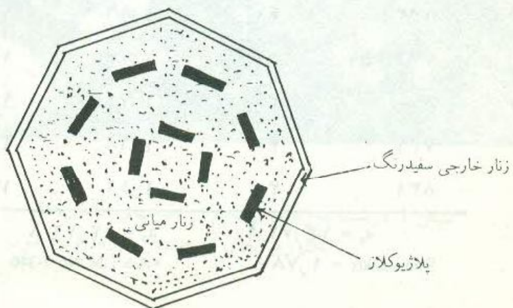
شکل ۳ مقطع یک بلور آنالسیم ۵/۱ سانتیمتری طالقان و وجود انکلوژیون - پلاژ - یوکلاز ( A_{pl}=44 ) به صورت هم مرکز در درون آن. شکل از روی مقطع ترسیم شده است.
