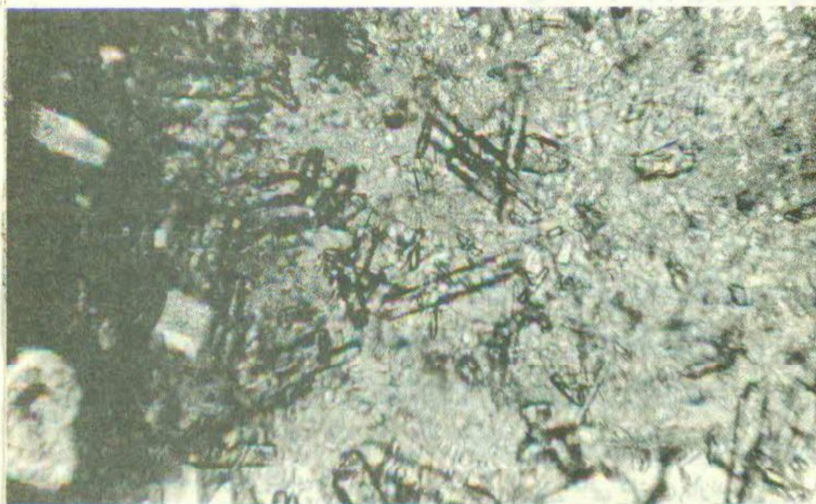
شکل ۱۰ سوزن های هیرستن در مرز بین بازالت (چپ) و زینولیت (راست) (x ۷۵).
