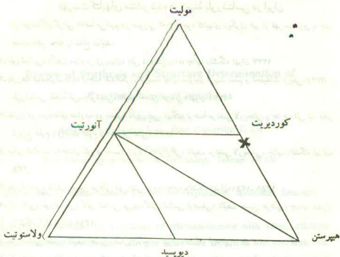
شکل ۱۱ نمودار ACF رخساره سانییدینیت.
