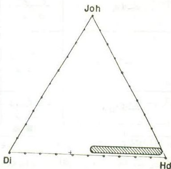
شکل ۳ ترکیب کانی شناختی پیروکسین های منطقه A'
