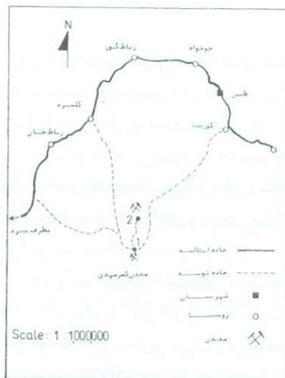
شکل ۱ موقعیت معدن فلوریت کمر مهدی و راههای ارتباطی آن.
