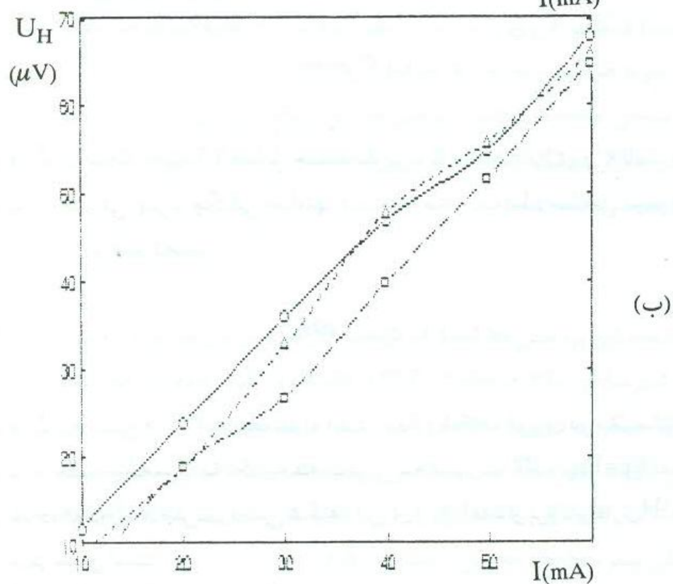
شکل ۲ نمودارهای ولتاژ هال به صورت تابعی از جریان طولی در میدان مغناطیسی ثابت B=400\text{ mT} (الف): در نمونه تک بلور PbTe (ب): برای سه نمونه بسبلور PbTe.
