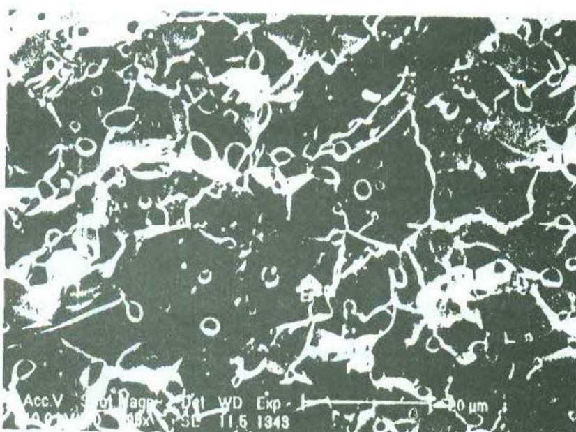
شکل ۳ تصویر میکروسکوپ الکترونی فریت نیکل با دمای تف‌جوشی ۱۵۰۰°C.
