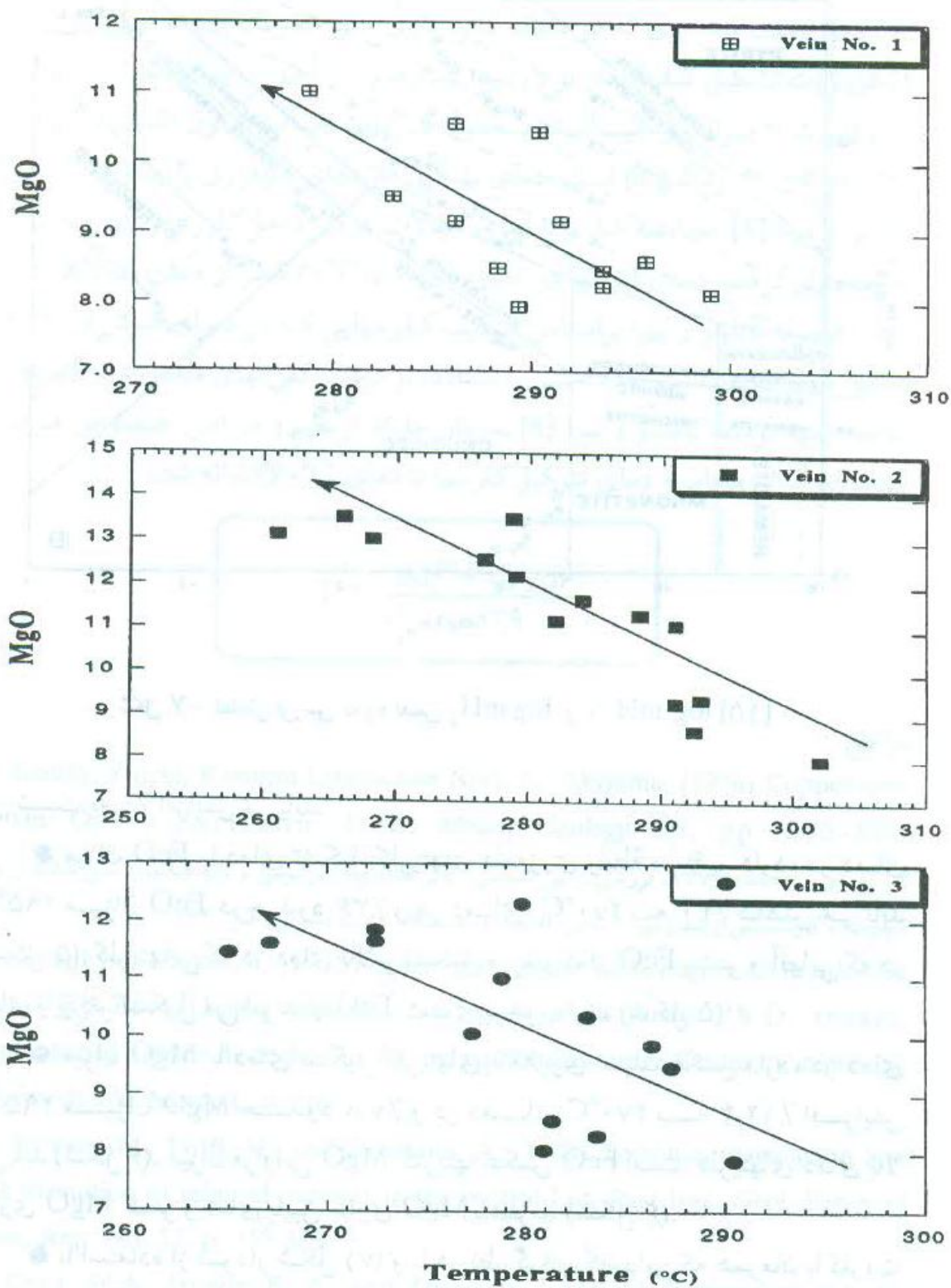
شکل ۶- نمایش بررسی نحوه تغییرات MgO و دما در کربنهای قلعه زری
