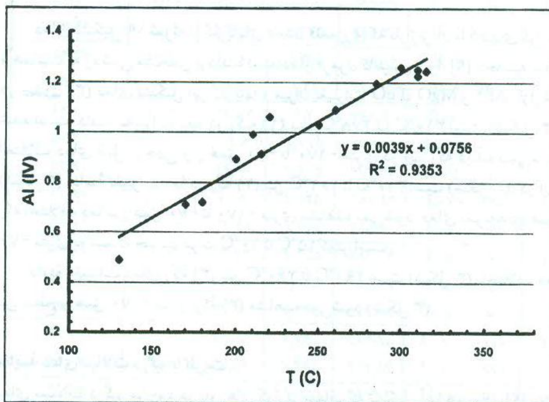
شکل ۴- نمایش بررسی میزان تغییرات Al (IV) و دما در کلریت‌های قلعه زری و کاتلینو و نیوا [۵] و ارائه معادله جدید جهت محاسبه دمای تشکیل کلریت
