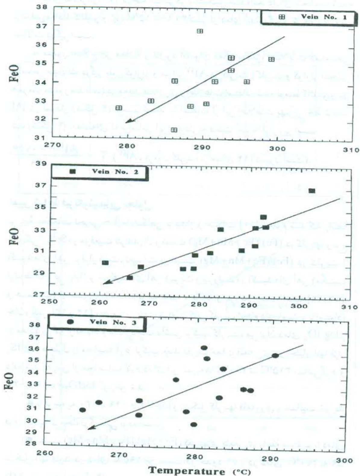
شکل ۵ - نمایش بررسی نحوه تغییرات FeO و دما در کالریتهای قلعه زری
