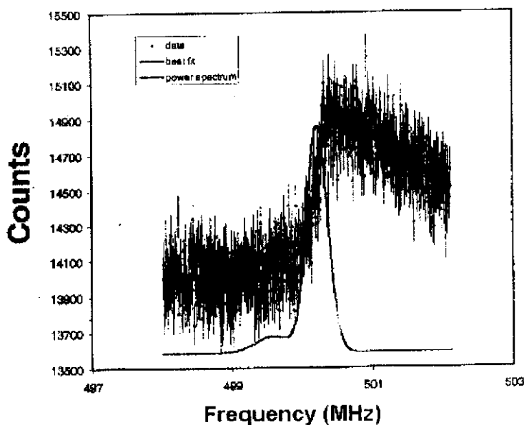
شکل ۱ - طیف NMRON مربوط به ^{54}\text{Mn} در نمونه بلوری \text{MnCl}_2 \cdot 4\text{H}_2\text{O} به ازای ۶٫۲ درصد کبالت، بسامد تشدید اصلی ۵۰۰٫۲۲MHz و خط اقماری، ۴۹۹٫۶ MHz است.
