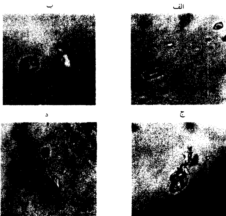
شکل ۶- آنکلوژیونهای اولیه تیپیک با ترکیب متفاوت در نمونه‌های مورد مطالعه
