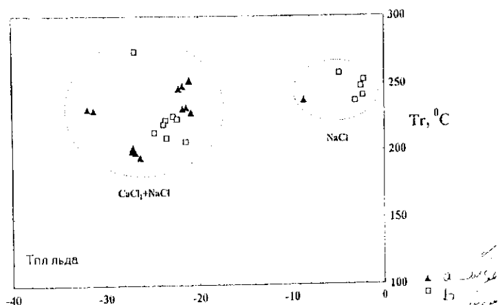
شکل ۷- نمودار رابطه دمای همگن ( Tr^{\circ}C ) و دمای ذوب یخ ( Tm ) در شاره های درگیر مطالعه شده در کانی کوارتز.
