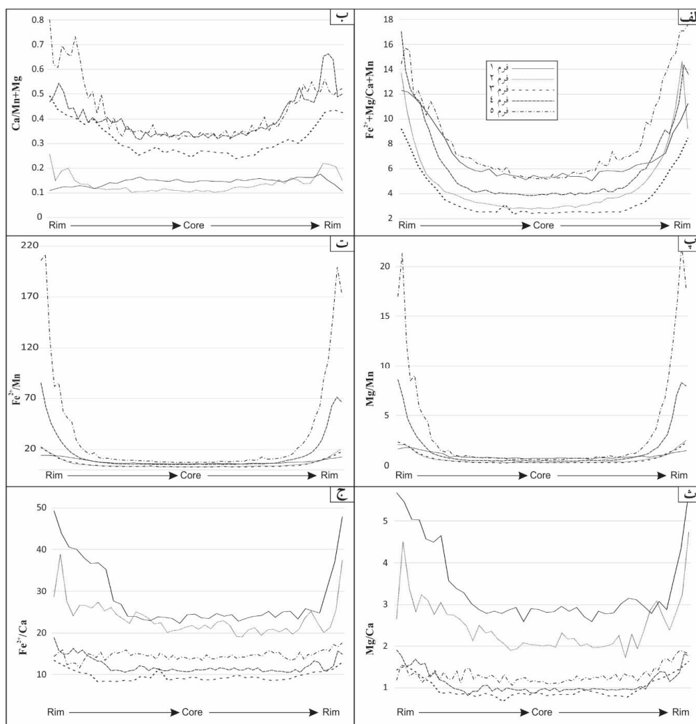
شکل ۵ تغییرات نسبت‌های کاتیونی از هسته تا حاشیه بلورها در فرم‌های مختلف گارنت در منطقه همدان؛ الف- (Fe^{2+}+Mg)/(Mn+Ca) ، ب- Ca/(Mn+Mg) ، پ- Mg/Mn ، ت- Fe^{2+}/Mn ، ج- Fe^{2+}/Ca ، ث- Mg/Ca .
