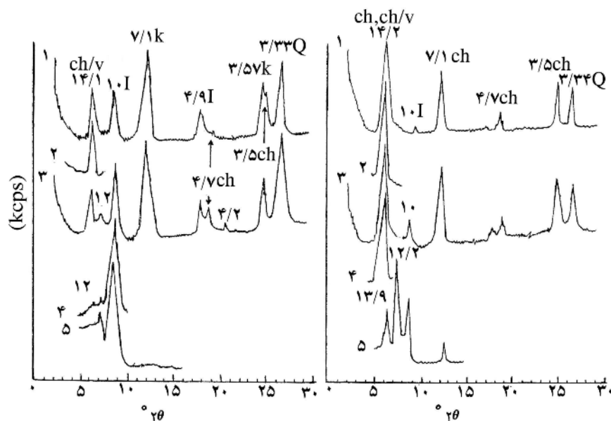
شکل ۱ پراش نگاشت پرتو ایکس ذرات رس افق A1 (۱۳-۰ نیمرخ خاک (۱). شکل ۲ پراش نگاشت پرتو ایکس ذرات رس افق C (۱۷۵-۱۲۲، نیمرخ خاک (۱). (آنالیز بعضی تیمارها (۲ و ۴ و ۵ در شکل ۱ و ۲) در زاویه محدود به 2\theta صورت گرفته است). پراش نگاشت ۱: نمونه اشباع شده با منیزیم پراش نگاشت ۲: نمونه ۱ + گلیکول پراش نگاشت ۳: نمونه اشباع شده با پتاسیم پراش نگاشت ۴: نمونه ۳ + دمای 350^\circ\text{C} به مدت ۲ ساعت پراش نگاشت ۵: نمونه ۳ + دمای 550^\circ\text{C} به مدت ۲ ساعت (اعداد روی قله ها به انگستروم) S = اسمکتیت I = ایلیت ch = کلریت Q = کوآرتز K = کائولینیت V = ورمیکولیت mi = میکا
