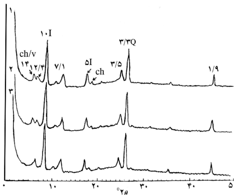
شکل ۳ پراش نگاشت پرتو ایکس از ذرات رس سنگ فیلایت هوازده (نیمرخ خاک (۱) پراش نگاشت ۱: نمونه اشباع شده با منیزیم. پراش نگاشت ۲: نمونه ۱ + گلیکول. پراش نگاشت ۳: نمونه اشباع با پتاسیم + دمای ۵۵۰ °C به مدت ۲ ساعت.
