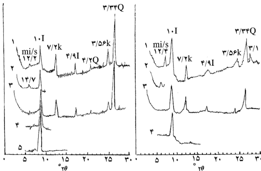
شکل ۶ پراش نگاشت پرتو ایکس ذرات رس
