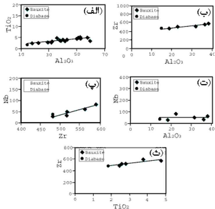
شکل ۶ نمودارهای همبستگی، الف) Al_2O_3 - TiO_2 ، ب) Al_2O_3 - Zr ، پ) Zr - Nb ، ت) Al_2O_3 - Nb ، ث) TiO_2 - Zr نمونه های بوکسیتی و سنگ دیاباز [۱۵]. خط پیوسته حاصل از درون یابی بهترین خط روند هوازدگی است.
