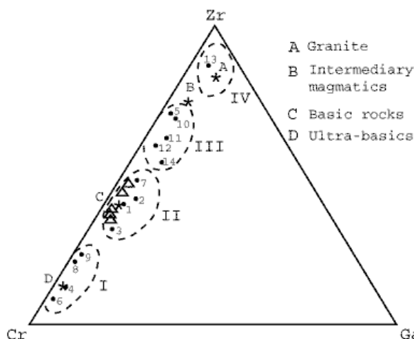
شکل ۴ محل نمونه‌های بوکسیت قپی (مثلث‌های توخالی) و مقایسه آن با بوکسیت‌های کارستی مدیترانه‌ای و بوکسیت لاتریتی ارکانزاس بر اساس مقادیر Ga, Cr, Zr آنها [۱۰]. به ترتیب بیانگر مناطق اثر سنگهای مادر الترامافیک، مافیک، حد واسط و اسیدی هستند. A, B, C, D (ستاره‌ها) به ترتیب مربوط به مقادیر عناصر Ga, Cr, Zr در سنگهای ماگمایی اسیدی، حد واسط، مافیک و الترامافیک می‌باشند. اعداد ۱ تا ۱۴ مربوط به ذخایر بوکسیتی مختلف در دنیا هستند که در جدول ۳ آورده شده‌اند.
