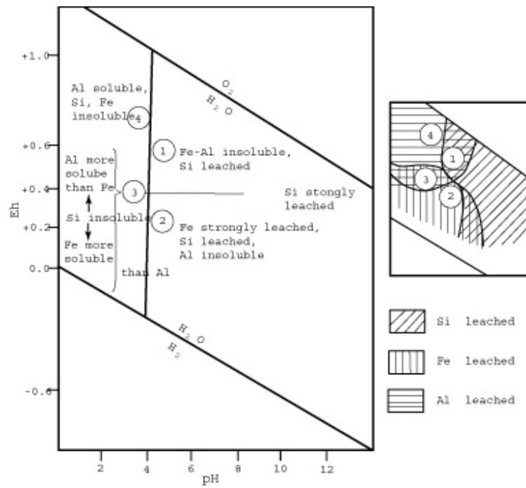
شکل ۷ نقش Eh و pH در تشکیل بوکسیت‌ها با توجه به تحرک عناصر [۱۸].
