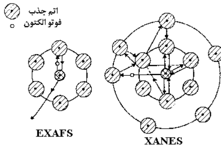
شکل ۱ نموداری از فرایند تکپراکنش در ناحیه EXAFS و نیز فرایند پراکنشهای متعدد در ناحیه XANES [۲].
