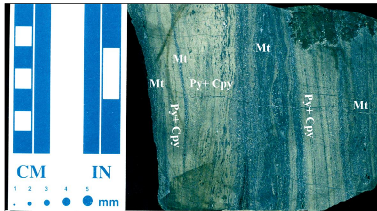
شکل ۶ کانی‌سازی لایه‌ای در نمونه دستی. لایه‌بندی در اثر تغییرات فراوانی کانیهای فلزی سولفیدی و اکسیدی ایجاد شده است.
