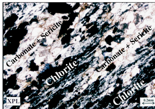
شکل ۴ کلریت شیست سازند تکنار.
