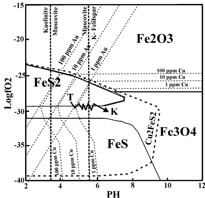
شکل ۱۶ نمودار \text{pH} - \log f\text{O}_2 در دمای T = 350^\circ\text{C} و سایر شرایطی که در نمودار مشخص شده است. مسیر مناسب TK برای کانسار تک I با توجه به پاراژنزه کانیها مشخص شده است که مسیری نسبتاً اکسیدان است [۱۱].
