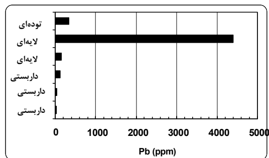
شکل ۱۱ تغییرات فراوانی سرب در بخش‌های مختلف کانی سازی تک I.
