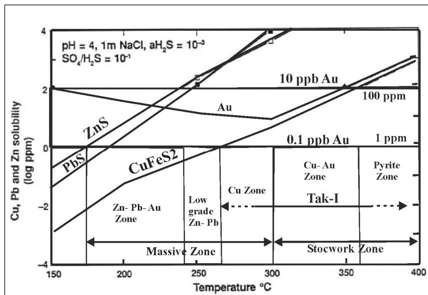
شکل ۱۵ نمودار بررسی وضعیت پایداری و نحوه ناپایدار شدن کمپلکس \text{Cu} ، \text{Au} ، \text{Pb} و \text{Zn} در شرایط \text{pH} = 4 و سایر موارد مشخص شده در شکل ۱۱. محدوده دمایی بخش داربستی و توده ای در کانسار ماسیوسولفید تک I ارائه شده است [۱۱].
