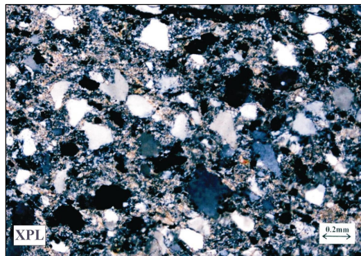
شکل ۳ تصویر میکروسکوپی از سرسیت شیست های سازند تکنار.
