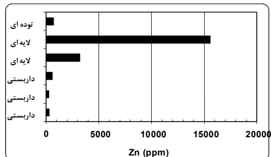
شکل ۱۰ تغییرات فراوانی روی در بخش‌های مختلف کانی سازی تک I.
