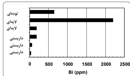
شکل ۱۴ تغییرات فراوانی بیسموت در بخش‌های مختلف کانی‌سازی تک I.
