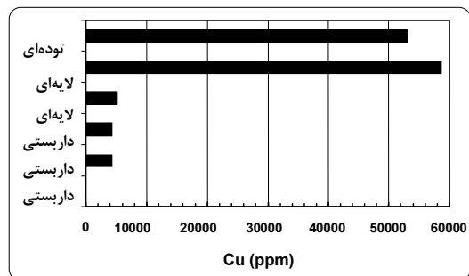
شکل ۹ تغییرات فراوانی مس در بخش‌های مختلف کانی سازی تک I.
