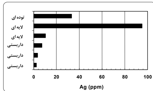
شکل ۱۳ تغییرات فراوانی نقره در بخش‌های مختلف کانی‌سازی تک I.
