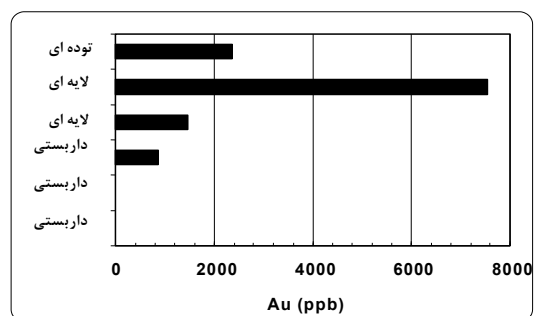
شکل ۱۲ تغییرات فراوانی طلا در بخش‌های مختلف کانی سازی تک I.
