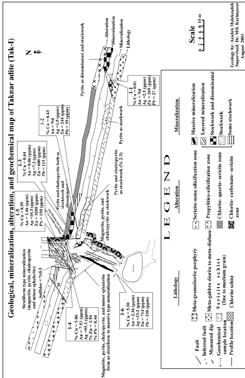
شکل ۵ نقشه زمین شناسی - کانی سازی - دگرسانی - ژئوشیمی تونل تک I [۱۱].
