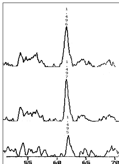
شکل ۸. قله شاخص اسمکتیت دی اکتاهدرال با فواصل لایه های (d=۰.۶۰) از d = ۱/۴۹۵ تا d = ۱/۴۹۷ به ترتیب از بالا به پایین مربوط به نمونه های Af99، Af56 و Af74 می باشد.
