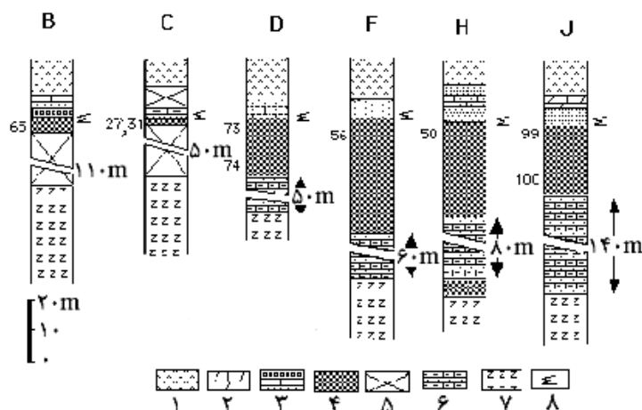
شکل ۲ نیمرخهای تهیه شده از سازندهای کُند زیرین و سمنان بالایی در منطقه شمال غرب افتر. ۱- ژپیس و ژپیس مارن دار، ۲- آهک دولومیت دار و یا دولومیت آهک دار، ۳- کنگلومرا، ماسه سنگ و آهک سلسنتین دار، ۴- بنتونیت، ۵- پوشش آلوویال، ۶- مارن‌های توفی سبز رنگ، همراه درون لایه‌هایی از ماسه و سیلت، ۷- زئولیت، ۸- بین انگشتی با ماسه سنگ، کنگلومرا و آهک سلسنتین دار. شماره‌های سمت چپ نیمرخ‌ها مربوط به شماره نمونه‌ها در متن مقاله است
