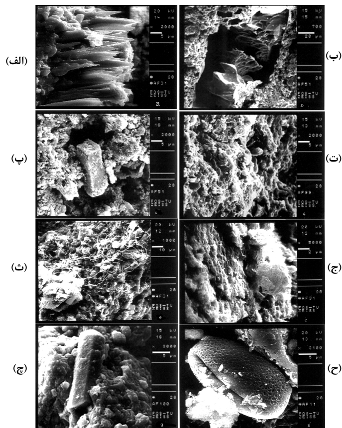
شکل ۹ الف) شیشه‌های شمشیری شکل، ب) انحلال تدریجی شیشه در مرکز و تشکیل اسمکتیت در اطراف آن، پ) تشکیل بلور در جازا ۲ در کنار اسمکتیتها، ت) تبدیل تدریجی شیشه به اسمکتیت از سمت راست به سمت چپ، ث) بدیل تدریجی اسمکتیت به موردنیت رشته‌ای شکل، ج) اسمکتیت لانه زنبوری و شیشه در سمت چپ و تبدیل بخشی از آن به اوپال در سمت راست، چ) یک بلور آپاتیت به همراه اسمکتیت‌های اطراف آن، ح) فسیل دیاتومه با پوسته سیلیسی. شماره نمونه‌ها، مقیاس و ضرایب بزرگ نمایی در حاشیه عکس‌ها ذکر شده‌اند.
