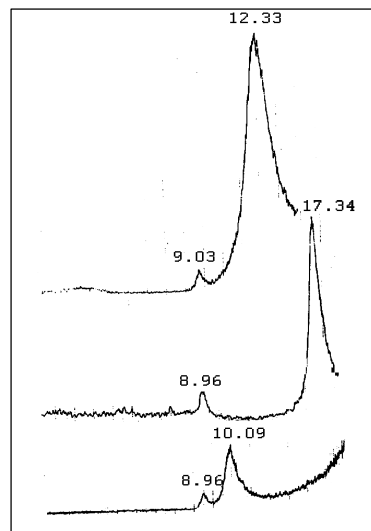
شکل ۷. طیف های XRD مربوط به اسمکتیت Af31 از نیمرخ C به ترتیب از بالا به پایین در شرایط عادی (d=۱۲/۳۳)، اتیلن گلیکولی شده (d = ۱۷/۳۴) و گرمادهی تا ۵۵۰ درجه سانتیگراد به مدت یک ساعت (d = ۱۰/۰۹). قله ظاهر شده در d = ۹/۰۳، d = ۸/۹۶ و d = ۸/۹۶ مربوط به آثار باقی مانده از کلینوپتیلولیت است که همراه رس باقی مانده است.
