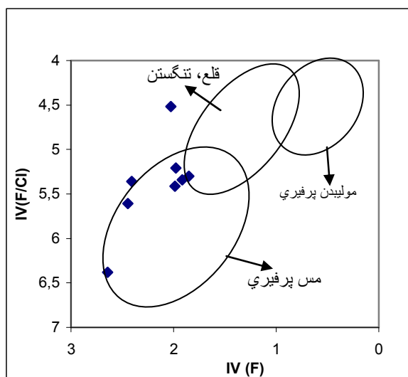
شکل ۸ مقادیر پیوندگاه F/Cl بیوتیت سنگ‌های گرانیتی زاهدان. گستره‌های مشخص شده در شکل برای کانسارهای مس پرفیری، مولین پرفیری و قلع و تنگستن از [۱]. نمونه‌های سنگ‌های گرانیتی زاهدان در گستره مس پرفیری و قلع قرار می‌گیرند.
