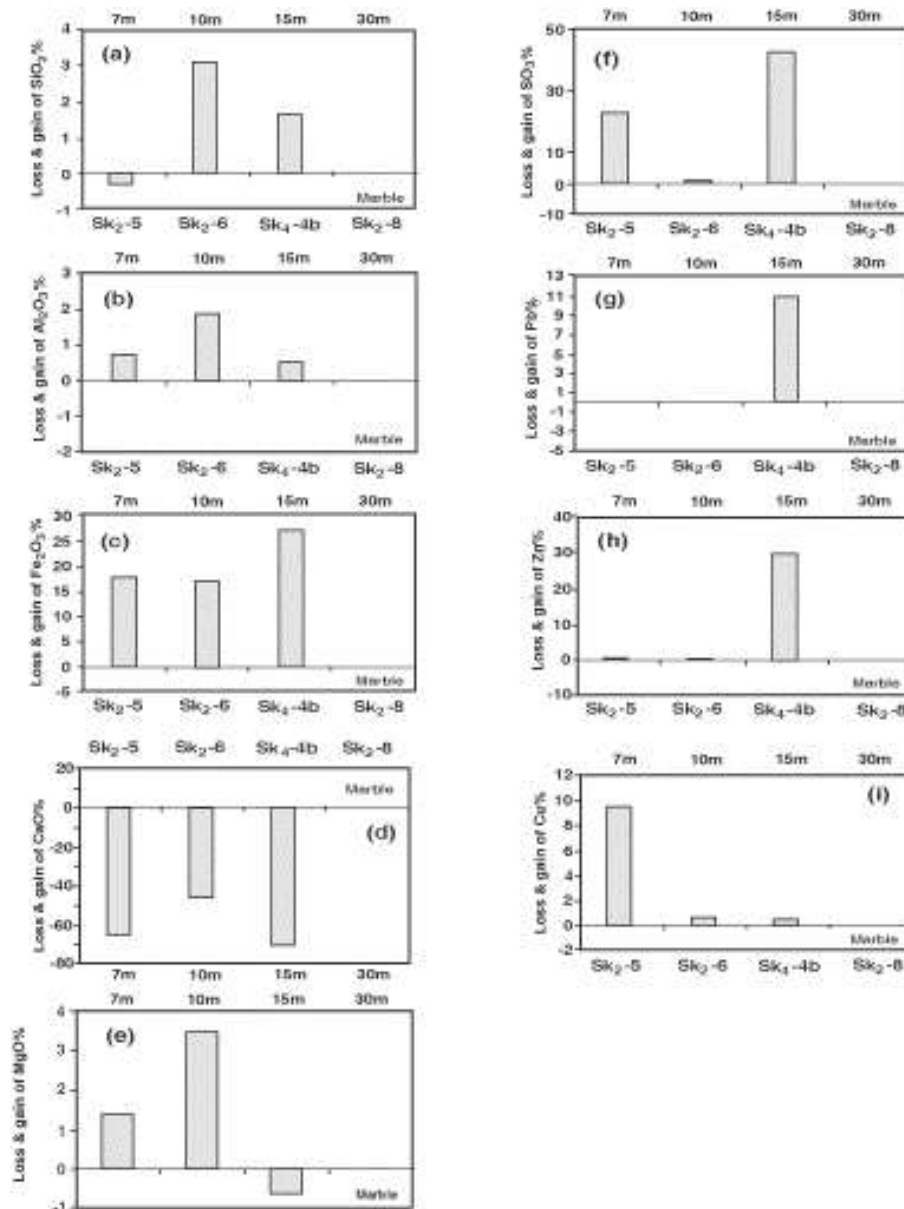
شکل ۲ تغییر جرم عناصر در نمونه‌های زون اسکارنی (دگرته‌ای) نسبت به مرمر (متامورفیک) دگرته‌د انشعابی) در طول مسیر SK 2 و SK 4 . (a) Si, (b) Al, (c) Fe, (d) Ca, (e) Mg, (f) S, (g) Pb, (h) Zn, (i) Cu
