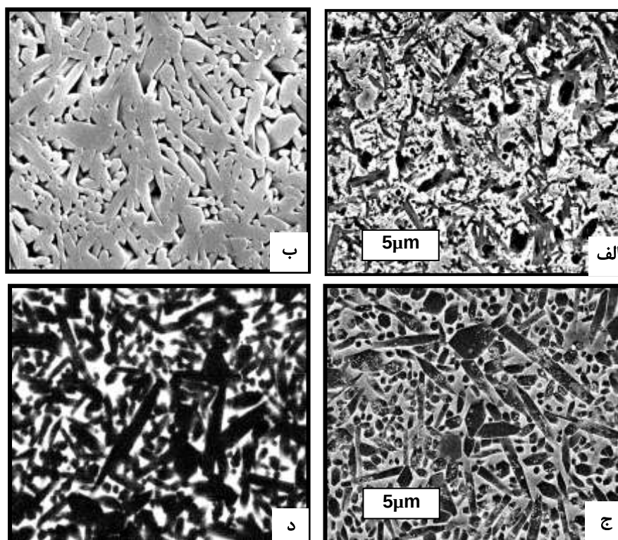
شکل ۴ انواع ریزساختارهای به دست آمده از نیتريد سيليسم در فرايندهای مختلف حکاکی الف: گرمایی در 1350^\circ\text{C} و به مدت ۳۰ دقیقه. ب: حکاکی شیمیایی با NaOH در دمای 350^\circ\text{C} به مدت ۵ دقیقه. ج: پلاسما با 15\% \text{O}_2 و 85\% \text{CF}_4 به مدت ۳۰ دقیقه. د: بدون فرایند حکاکی و مشاهده به روش SE.
