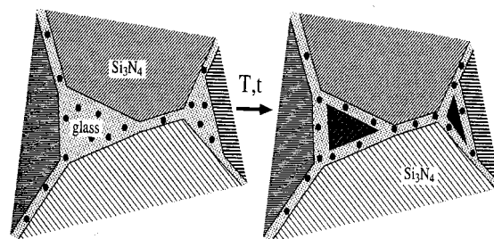
شکل ۸ ریز ساختار شماتیکی نیتريد سيليسيم كه در آن فاز بين دانه‌ای به خوبی مشخص شده است.
