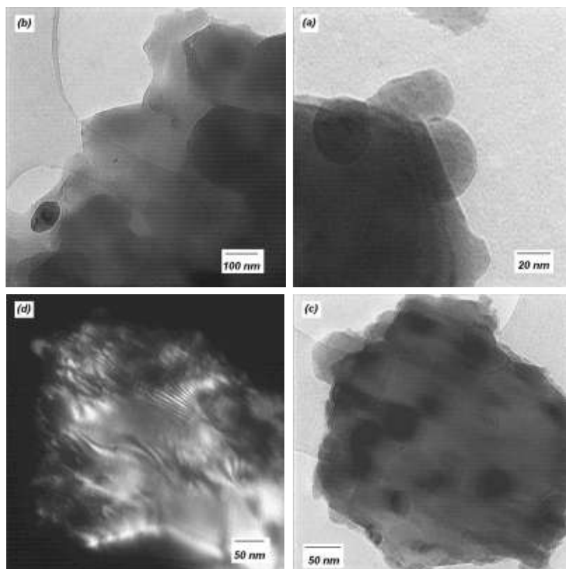
شکل ۹ تصاویر میکروسکوپ الکترونی تراگسیلی از ذرات مختلف پودر آسیاب شده به مدت ۲۴ ساعت که سیر تحول تدریجی آمیخته شدن ذرات Al و SiC را نشان می دهند. تصویر a: ذرات شبه کروی Al بر سطح ذرات لبه دار SiC، تصویر b: مرحله اولیه استتار ذرات SiC توسط Al، تصویر c: توزیع تقریباً همگن ذرات SiC در Al، تصویر d: تصویر منطقه تاریک از لایه های Al بر روی ذرات SiC.
