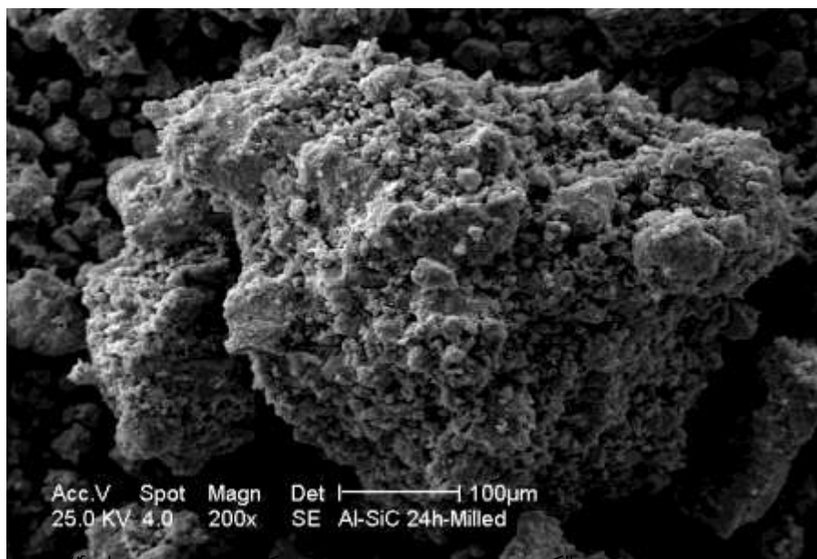
شکل ۳- تصویر میکروسکوپ الکترونی روبشی یک ذره آلومینیم کلوه‌ای شده پس از ۲۴ ساعت آسیاب‌کاری.
