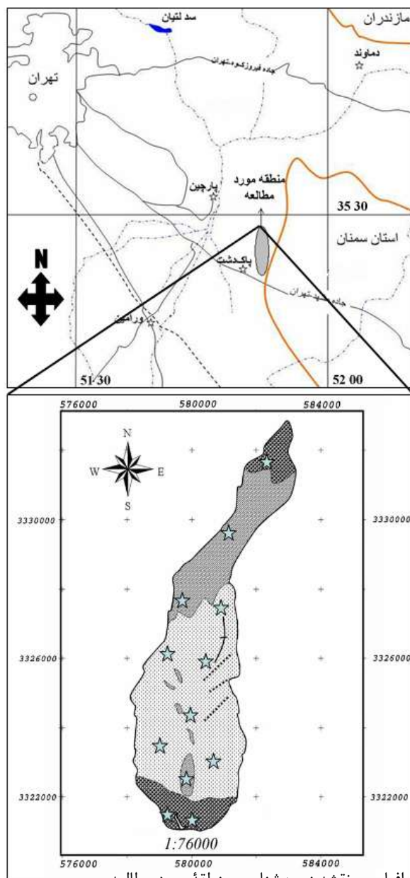
شکل ۱ موقعیت جغرافیایی و نقشه زمین‌شناسی منطقه مورد مطالعه.
