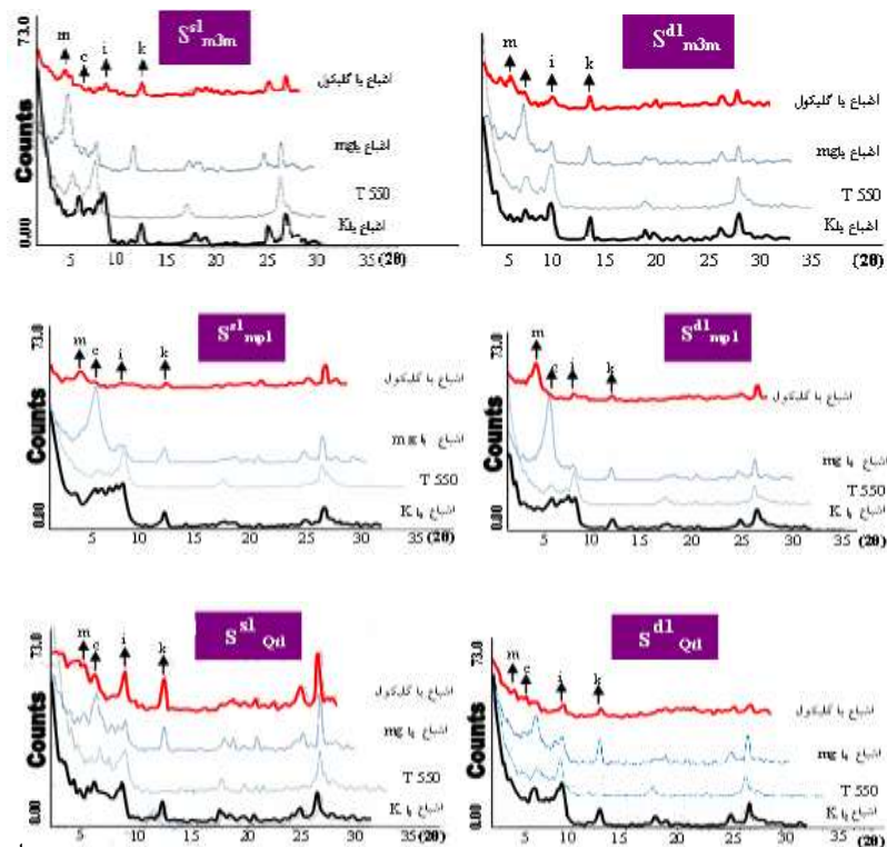
شکل ۲ نمونه‌ای از سایج آزمایش پراس پرو ایس واحد های سنی حوضه ابجیز لا نشور. نمودارهای سمت چپ مربوط به نمونه های سطحی و نمودارهای سمت راست مربوط به نمونه های آبراه های است که در آنها (m) مونت مورینیت، (c) کلریت، (i) ایلیت و (k) کائولینیت است. الف) واحدهای سرخ نشوژن، ب) سازند هزار دره و ج) آبرفت های کواترنر. علائم موجود در هر نمودار در جدول ۱ توضیح داده شد.
