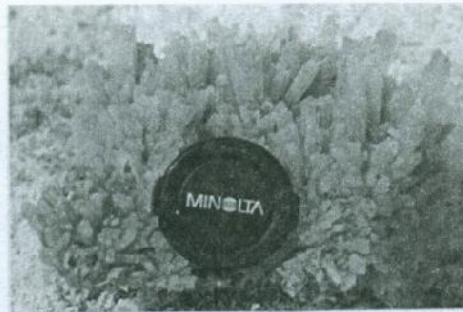
شکل ۶ بلور های ژپس با ماکل دم پرستویی در کویر سیاه کوه.
