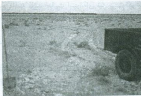
شکل ۱۳ لایه سولفات سدیم در سطح زمین در شرق مزرعه علی آباد در کویر سیاه کوه. اثر فرورفتگی چرخ خودرو در این نوع زمینها که شبیه مناطق پوشیده از برف هستند دیده می شود.
