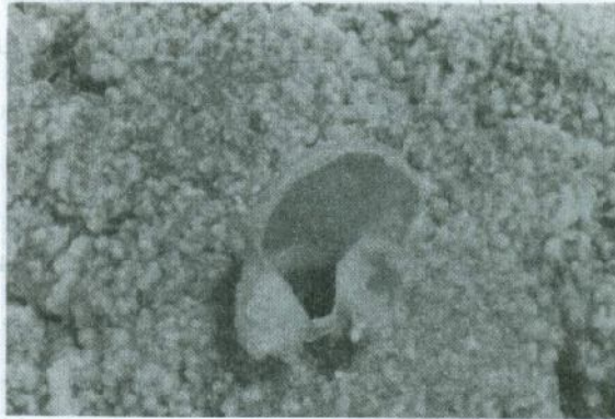
شکل ۸. هالیت استوانه ای در کویر سیاه کوه.
