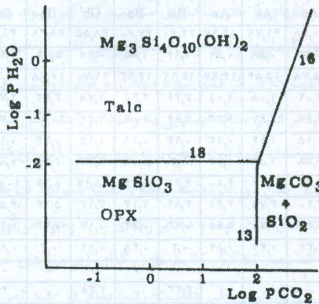
شکل ۱۹ سیستم \text{MgO} - \text{SiO}_2 - \text{CO}_2 - \text{H}_2\text{O} ، t = 327^\circ\text{C} ، \text{MgO}:\text{SiO}_2 = 3:4
