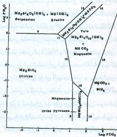
شکل ۱۸ سیستم \text{MgO} - \text{SiO}_2 - \text{CO}_2 - \text{H}_2\text{O} ، t = 327^\circ\text{C} ، \text{MgO}:\text{SiO}_2 = 2:1
