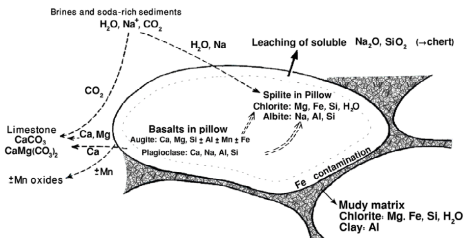
شکل ۱۱ تبادلهایی که هنگام اسپیلیتی شدن گدازه‌های بالشی رخ می‌دهند (برگرفته از [۳۸]).
