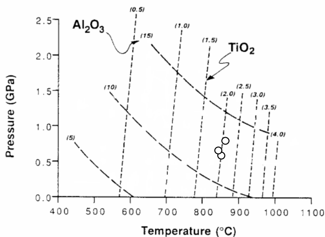
شکل ۱۲ ایزوپلت‌های \text{Al}_2\text{O}_3 و \text{TiO}_2 کلسیم آمفیبول‌ها بر پایه درصد وزنی به عنوان تابعی برای تعیین فشار و دما [۳۰] و موقعیت نمونه‌های مورد مطالعه بر روی آن.
