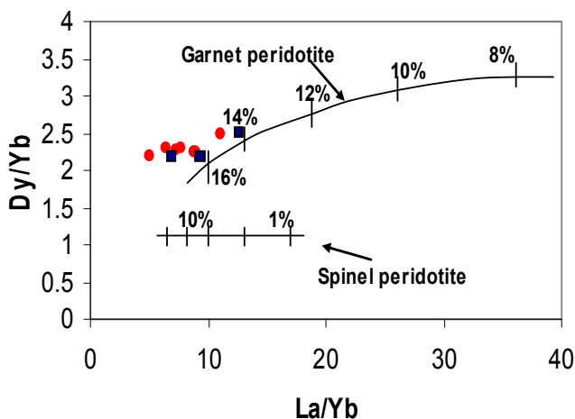
شکل ۱۱ الف) نمودار تعیین درجه ذوب بخشی محل منشأ ماگمای تشکیل دهنده سنگهای منطقه مورد مطالعه (اقتباس از [۳۴]). ب) نمودار تعیین مدل ذوب بخشی تعادلی در گوشته غنی‌شده و NMORB برای نمونه‌ای منطقه بر اساس مقادیر [۲۱].
