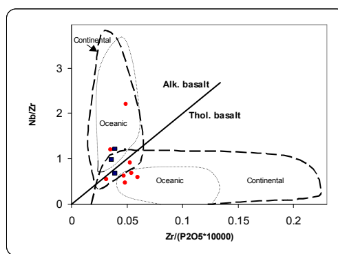
شکل ۵ تعیین سری ماگمایی سنگهای آذرین منطقه مورد مطالعه با استفاده از نمودارهای متمایز کننده الف) از [۱۳]، ب) از [۱۴]، ج) از [۱۵]، د) از [۱۶].
