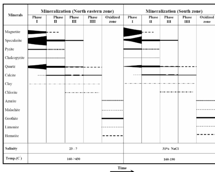
شکل ۴ دنباله پارائزی زونهای کانی‌سازی آهن.
