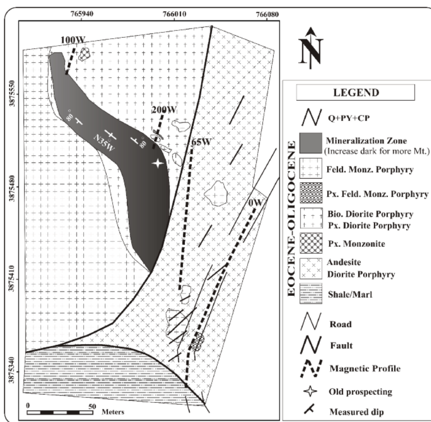
شکل ۲ زمین‌شناسی گستره زون جنوبی.
