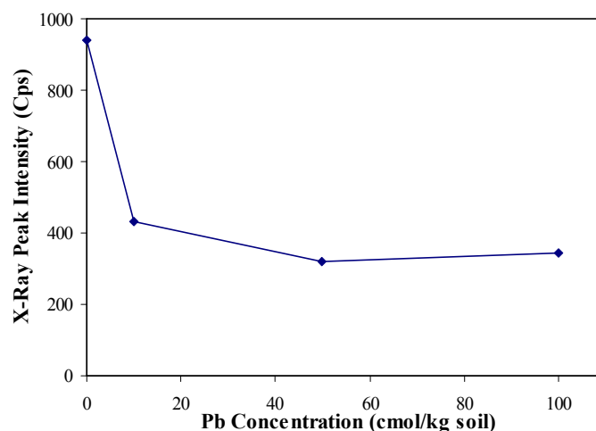
شکل ۹ تغییرات شدت قله اصلی ( \text{Å} ۷/۱) در کانی کائولینیت ناشی از افزایش غلظت آلاینده سرب
