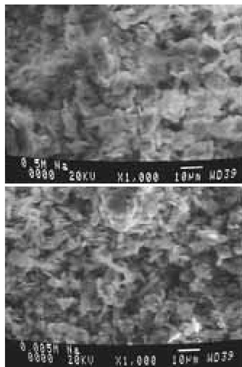
شکل ۳ نیمرخ عرضی نمونه کائولینیت با غلظت‌های ۰/۰۰۵ و ۰/۵ مولار کاتیون تک ظرفیتی سدیم؛ بزرگ‌نمایی ۱۰۰۰ برابر.
